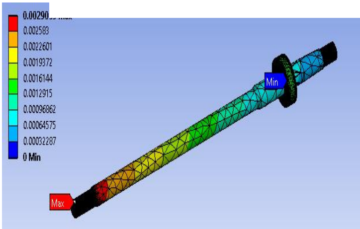
टॉर्शन में एक्सल बीम की ताकत का विश्लेषण
