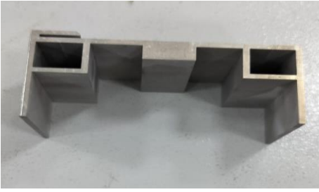
एक्सट्रूजन डाई नमूने के लिए वायरकट प्रोफाइल मशीनीकरण
